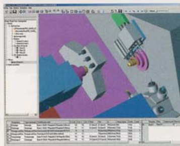
Simulation réelle d'une décolleteuse
