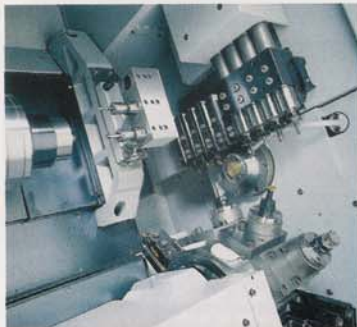
Type de MOCN pilotée par SylvieXpert
